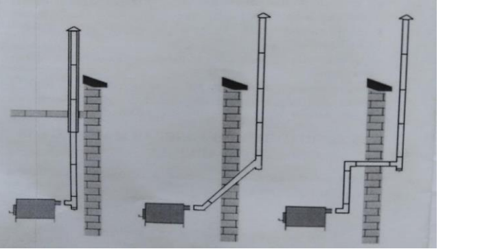
Рисунок 2. Варианты конфигурации дымохода
