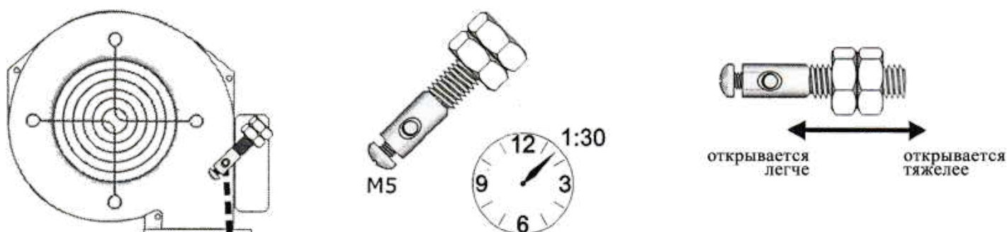
Регулировка контргруза на вентиляторе (рис. 3)
