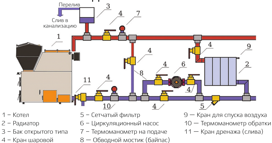
Рис. 6. Схема подключения котла к 2-х трубной открытой системе с принудительной циркуляцией теплоносителя
