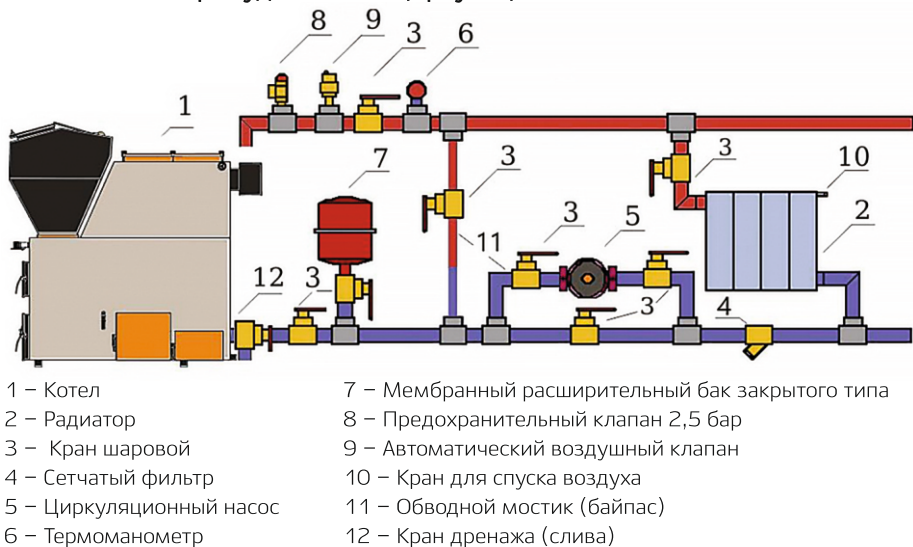
Рис. 7. Схема подключения котла к 2-х трубной закрытой системе с принудительной циркуляцией теплоносителя
