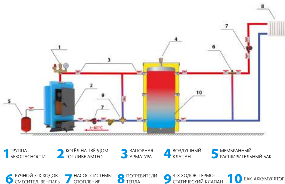
Рисунок 2(а). Типовая схема обвязки котла Amteo с баком-аккумулятором
