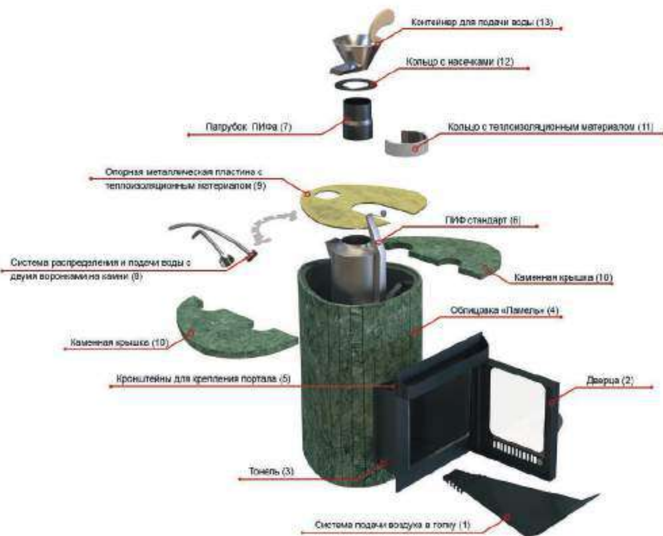
Рис. № 11 Схема установки ПИФ на печь
