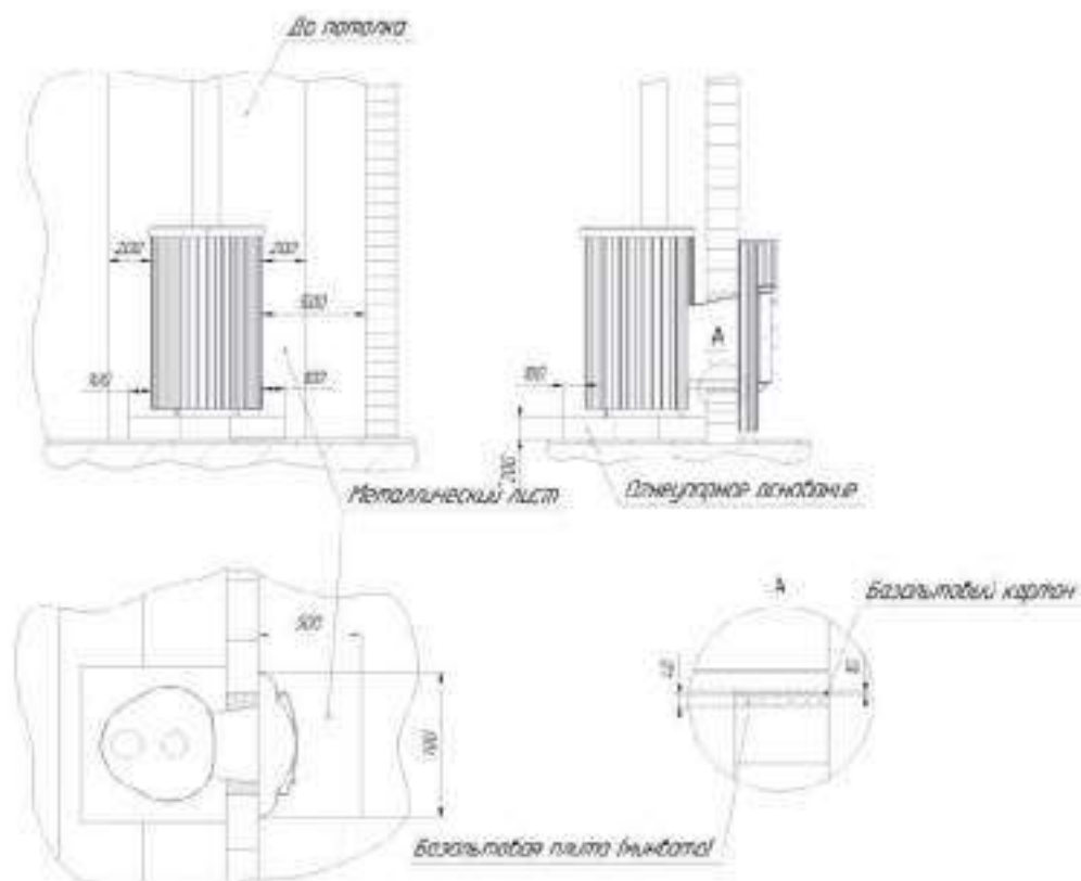
Рис.№ 3 Схема установки банной печи «Мини», «Малютка», «Оптим», «Квадра», «Макси» (серии ПФ) на минимально безопасном расстоянии от несущих и ограждающих конструкций.
