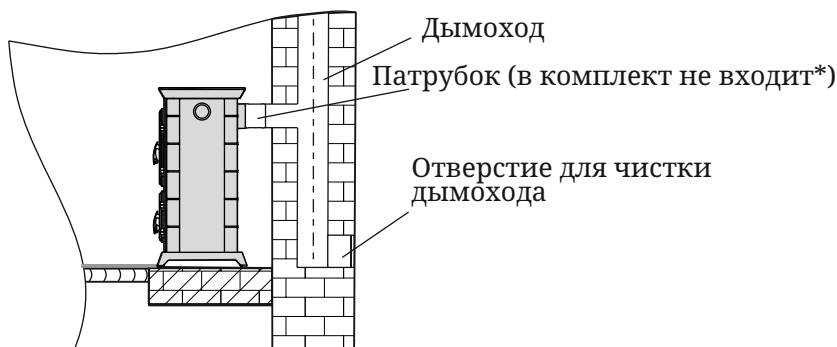
Рисунок 6. Схема присоединения печи к стационарному дымоходу из кирпича в помещении из негорючего материала
