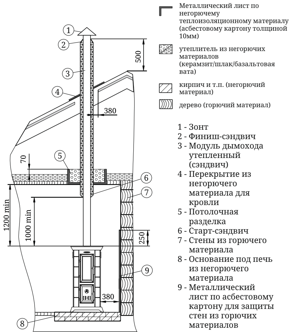
Рисунок 7. Пример монтажа печи «Статика Тетра» с присоединением к металлическому дымоходу
